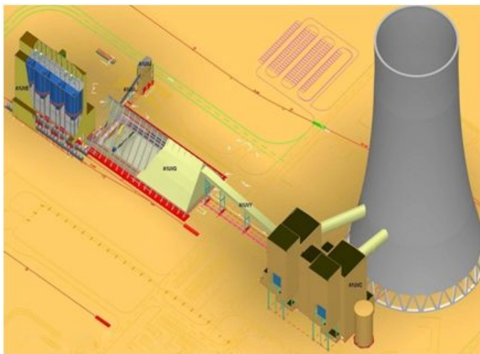
instalacja odsiarczania spalin
