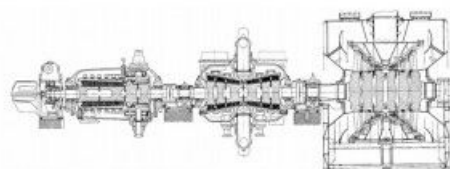
przekrój turbiny
