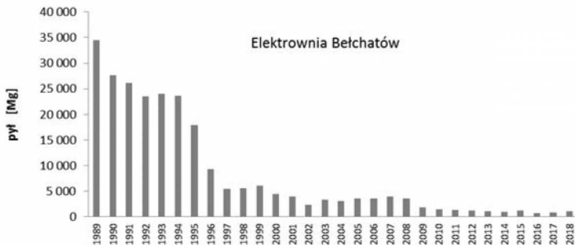
Wyk. Redukcja emisji pyłów na przestrzeni lat w Elektrowni Bełchatów.
